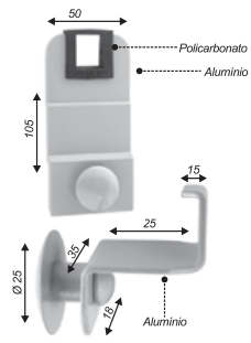
Conjunto acessório V/V para 1587
