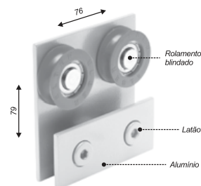
Carrinho duplo 2 furos para AP-68 (portas até 80kg)
