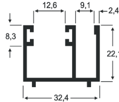
AP - 45 0,357 Kg/m
