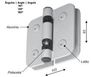
Dobradiça automática dupla
