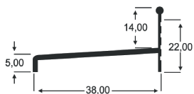
AP - 460 0,189 Kg/m
