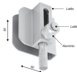
Trinco de pressão para janela de correr
