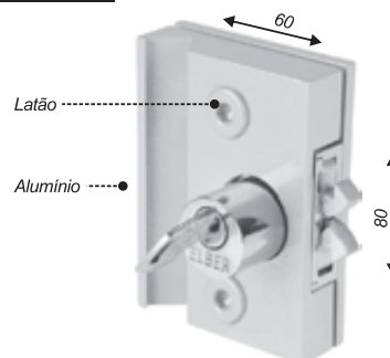
Minifechadura direita reforçada p/ janela de correr
