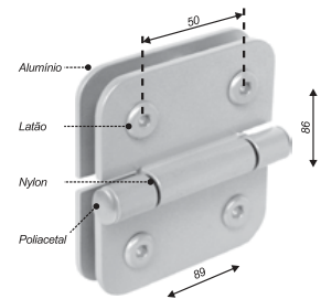
Dobradiça MAXIM-AR V/V (50mm entre furos)
