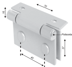
Dobraçã MAXIM-AR V/A (40mm entre furos)
