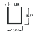
AP - 12 0,173 Kg/m
