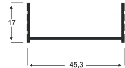
AP - 156 0,184 Kg/m
