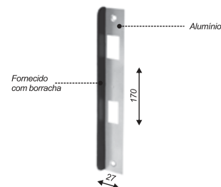
Batedeira em alvenaria para 1520TA
