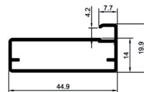
AP-907 0,409 Kg/m
