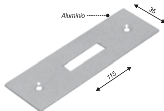
Testeira para 1510X e 1520X no piso
