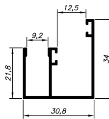
AP - 140 0,365 Kg/m
