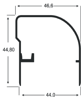
AP - 54 0,450 Kg/m
