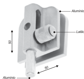
Trinco com ferrolho lateral
