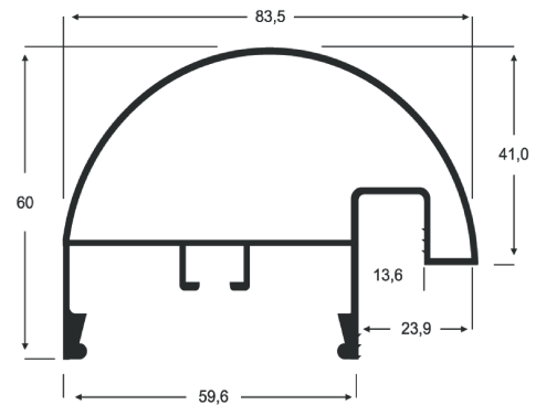
AP - 84 1,098 Kg/m
