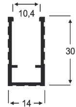
AP - 158 0,192 Kg/m
