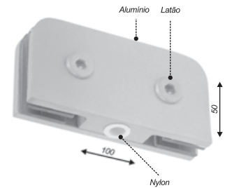
Dobradiça pino para basculante 50x100mm
