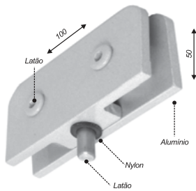
Dobradiça pino para basculante 50x100mm
