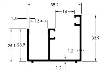
AP - 141 0,458 Kg/m
