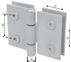
Dobraçã MAXIM-AR V/V (40mm entre furos)
