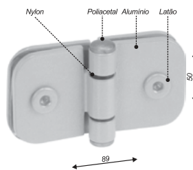
Dobradiça dupla pequena para janela
