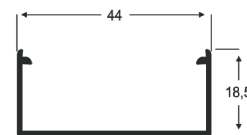
AP - 79 0,316 Kg/m
