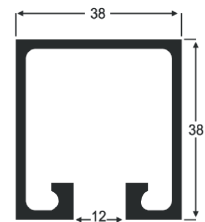
AP - 37 0,728 Kg/m
