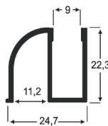
AP - 62 0,236 Kg/m
