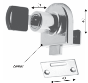
Fechadura de pressão com lingueta para rock
