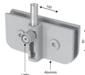
Trinco inferior sem núcleo 50x100mm (NOVO MODELO)
