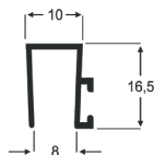
AP - 15 0,166 Kg/m
