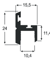
AP - 17 0,260 Kg/m
