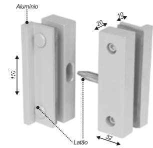
Conjunto mão de amigo para portas de correr com sistema deslizante
