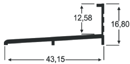
AP - 153 0,173 Kg/m
