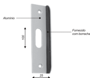
Batedeira em alvenaria para 1520
