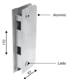
Contra-fechadura sem maçaneta (Vidro fixo) p/ 1520TA
