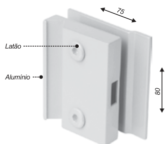
Contrafechadura V/V para 1510/22
