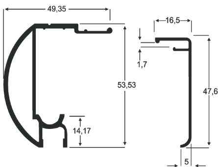
AP - 60A 0,717 Kg/m
