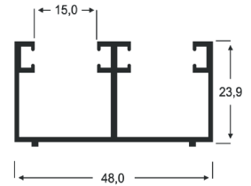
AP - 39 0,522 Kg/m
