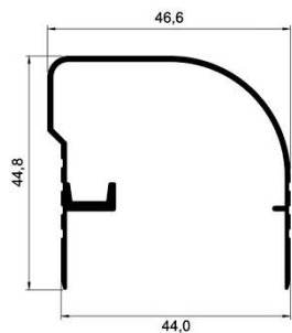
AP - 86 0,447 Kg/m
