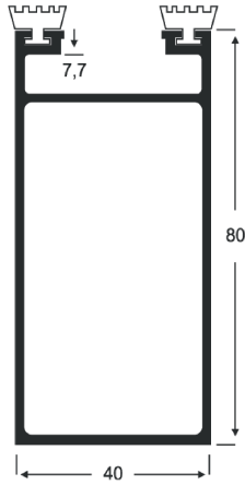
AP - 36 1,207 Kg/m
