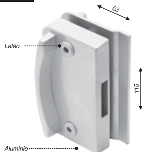
Contra-fechadura V/V para 1510X
