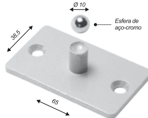
Pivô inferior em inox para 1102
