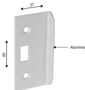
Batedeira V/A para 1510/22
