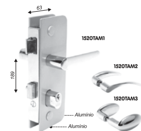
Fechadura de centro para maçaneta com 2 cilindros
