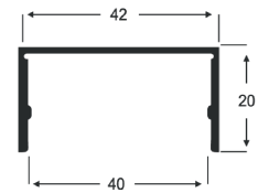
AP - 34 0,241 Kg/m
