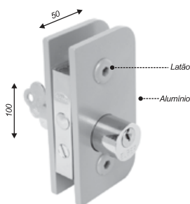
Fechadura de centro com 2 cilindros
