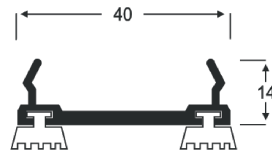
AP - 35 0,376 Kg/m
