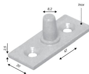
Pivô em inox para 1101, 1230 e 1231
