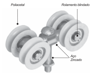
Roldana quádrupla para trilho AP-68
