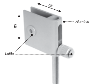
Trinco para janela de correr
