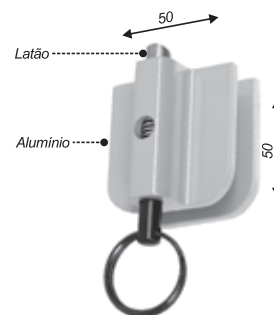
Trinco central para basculante com adaptador para corrente + 2 argolas
