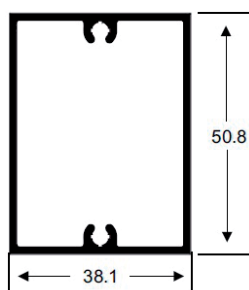
CG - 104 0,802 Kg/m
