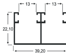
AP - 38 0,391 Kg/m
