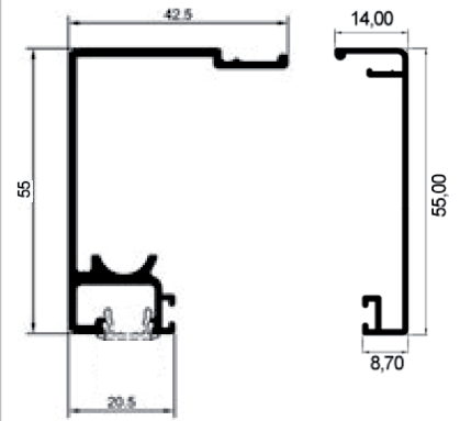
AP - 49A 0,650 Kg/m
