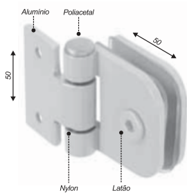
Dobradiça simples pequena para janela
