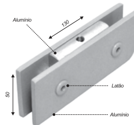
Suporte de canto com rosca para roldana 1150
