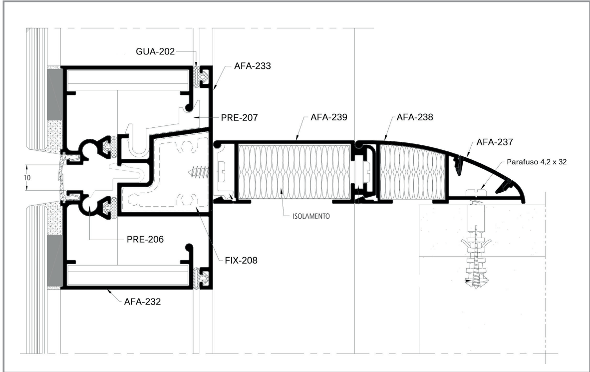
CORTE 08
