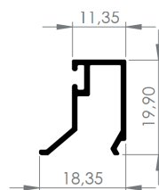
AP27 BAGUETE 0,237 Kg/m
