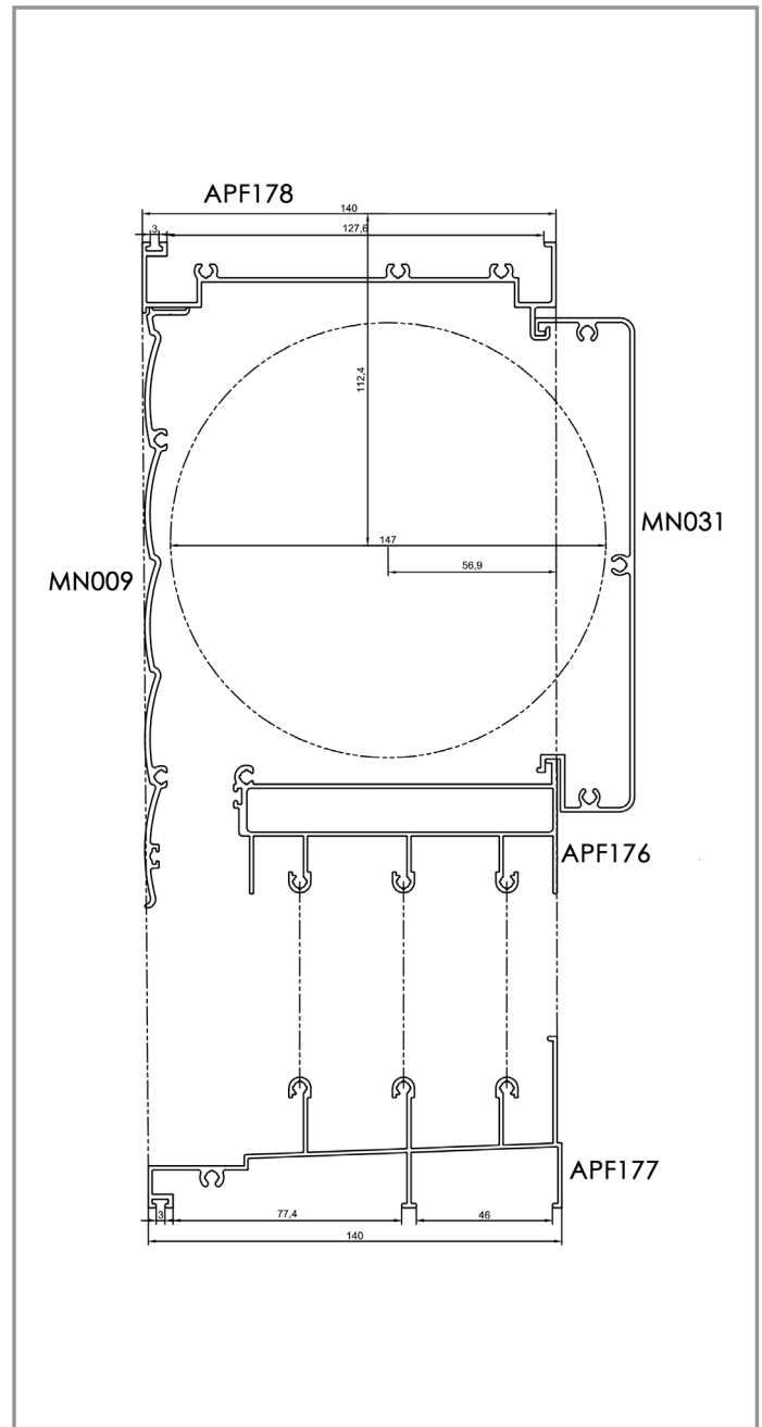
JANELA INTEGRADA 3 FOLHAS
