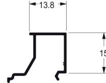
SU103 0,133 Kg/m BAGUETE
