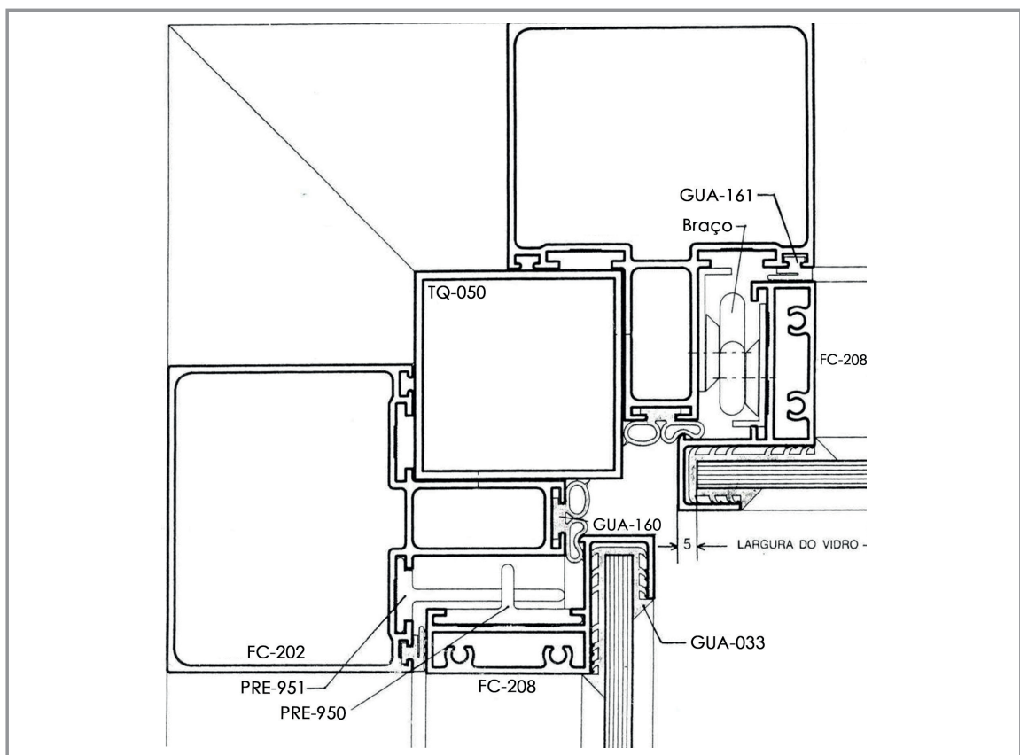
CORTE 04
