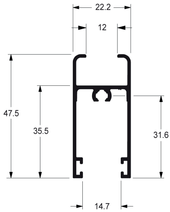
SU186 0,445 Kg/m TRAVESSA DA FOLHA
