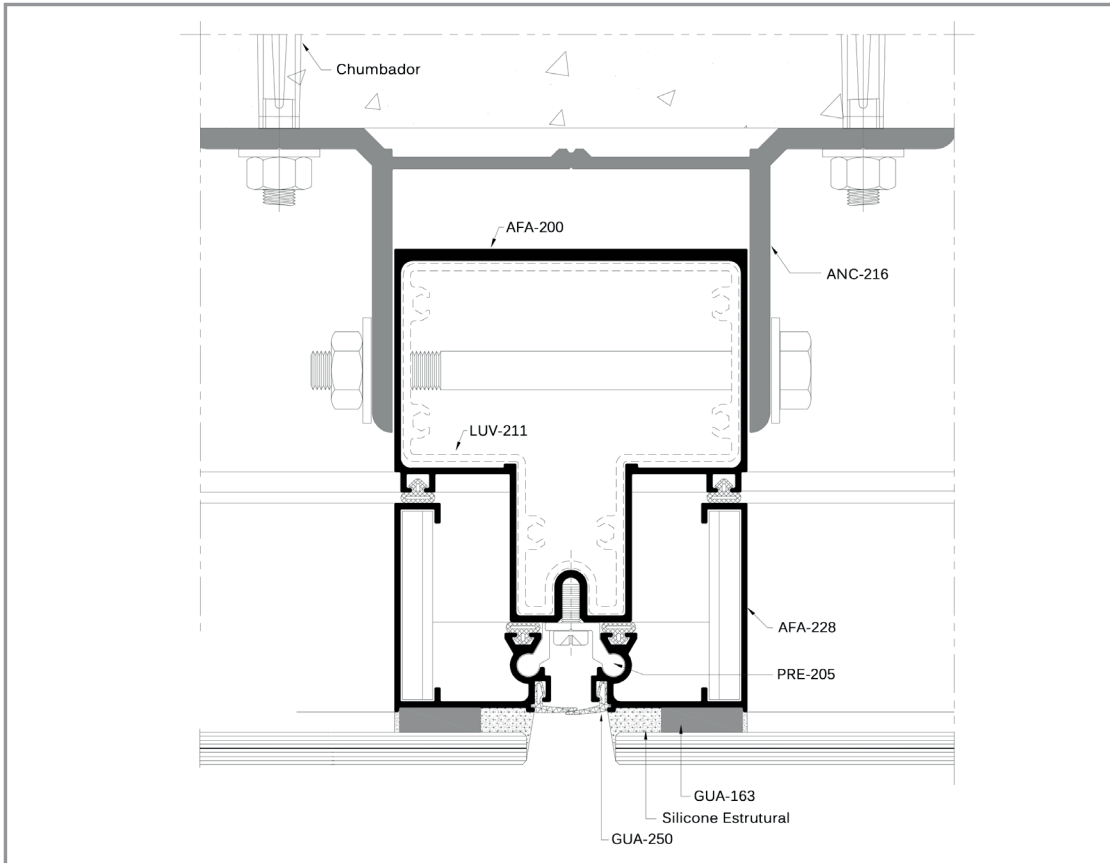
CORTE 02
