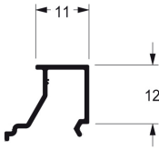
SU102 0,110 Kg/m BAGUETE
