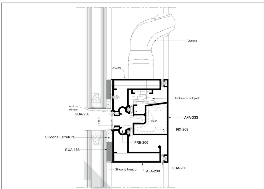
CORTE 04
