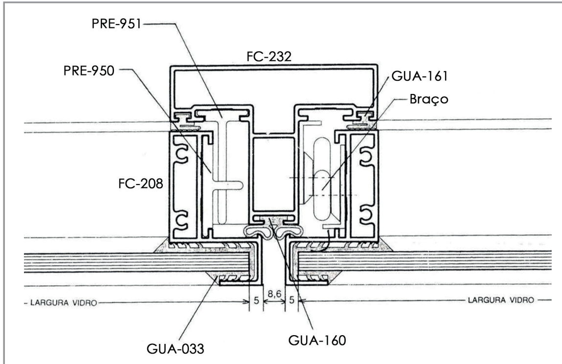
CORTE 06
