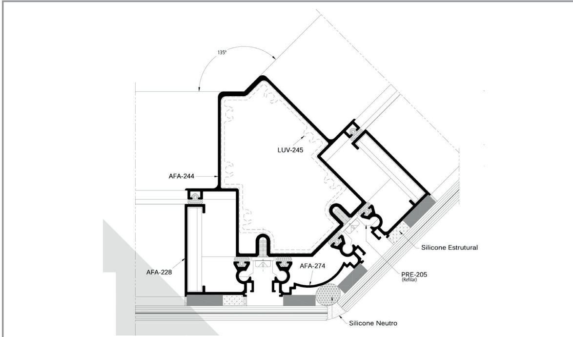
CORTE 06
