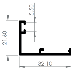
AP26 CANTONEIRA 0,237 Kg/m
