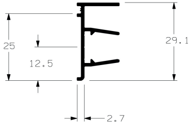
SU008 0,178 Kg/m COMPLEMENTO MARCO LATERAL
