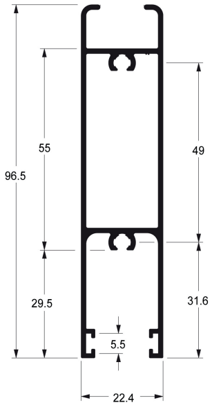
SU226 0,922 Kg/m TRAVESSA INFERIOR SEM BAGUETE
