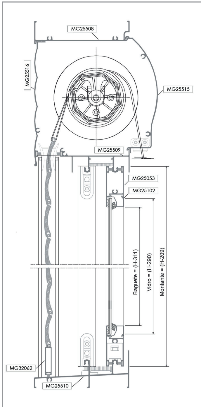
JANELA INTEGRADA 2 FOLHAS
