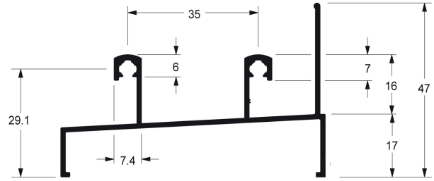
SU002 TRILHO INFERIOR JANELA 2 PLANOS
