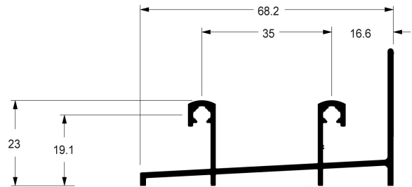
SU228 TRILHO INFERIOR PORTA 2 PLANOS
