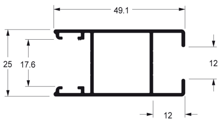
SU055 0,501 Kg/m MONTANTE SEM BAGUETE
