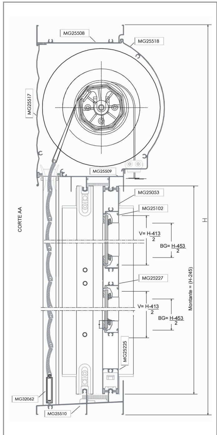
PORTA INTEGRADA 2 FOLHAS
