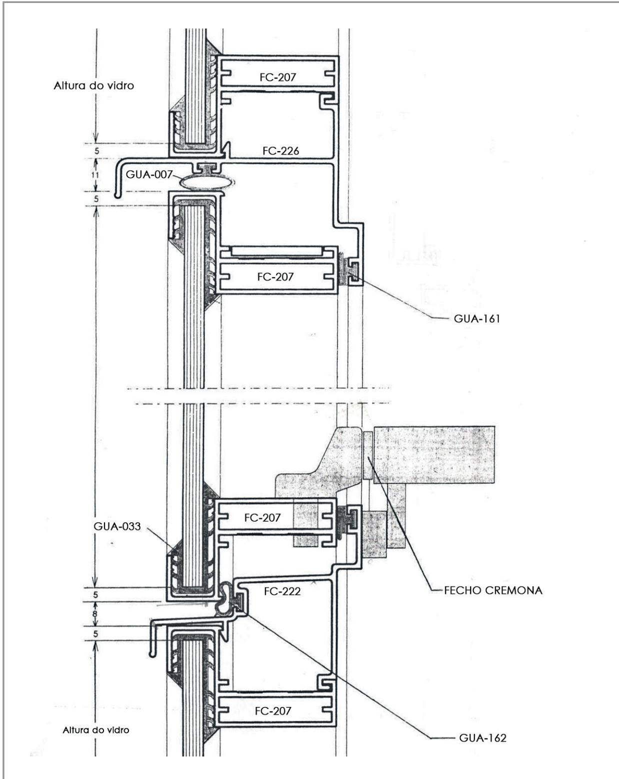
CORTE 05
