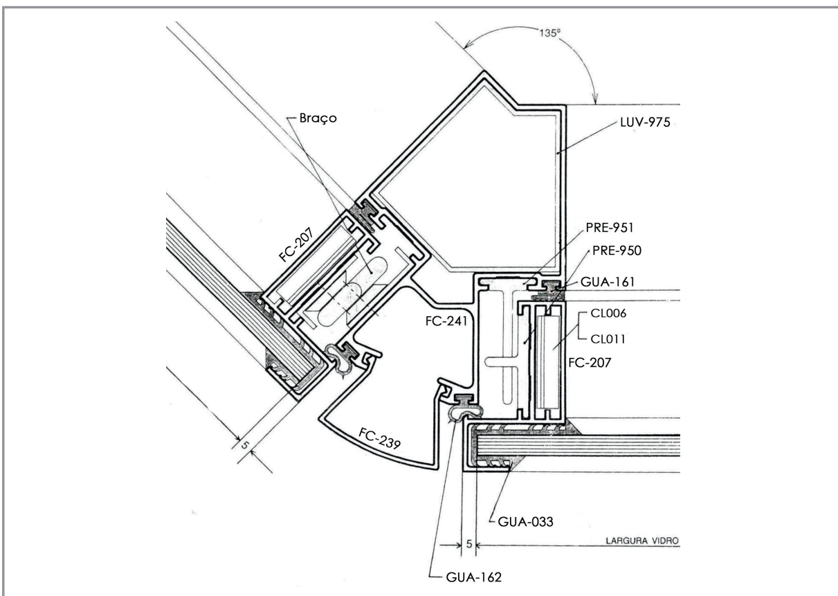
CORTE 02
