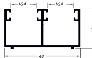
AP39 TRILHO INFERIOR DUPLO 10mm 0,512 Kg/m
