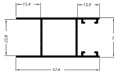
SU068 0,491 Kg/m MONTANTE DA FOLHA VENEZIANA
