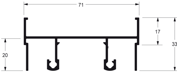
SU001 TRILHO SUPERIOR 2 PLANOS
