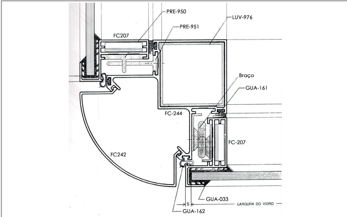
CORTE 02
