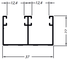
AP38 TRILHO INFERIOR DUPLO 08mm 0,316 Kg/m
