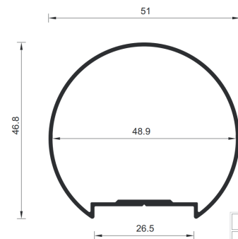
AP71 0,487 Kg/m SUPERIOR REDONDO
