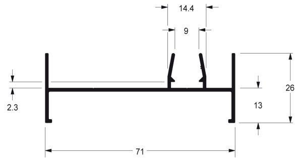
SU003 MARCO LATERAL 2 PLANOS
