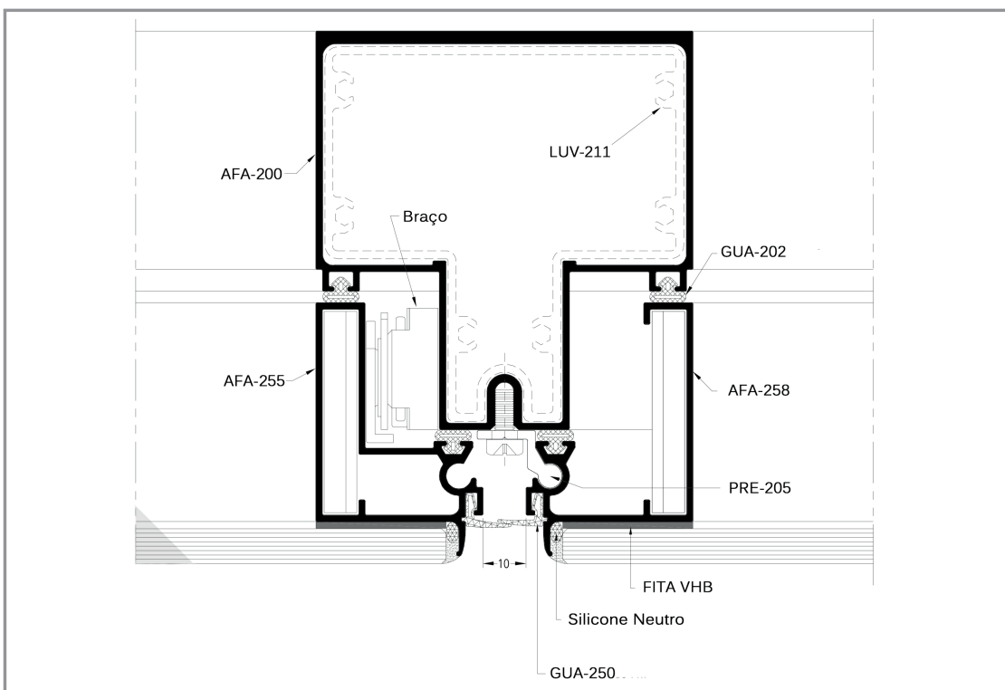
CORTE 02
