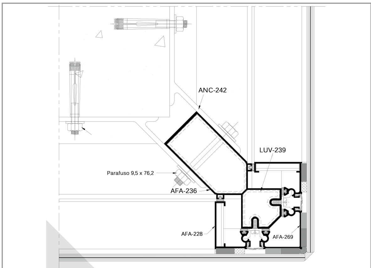
CORTE 08
