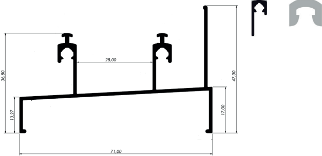
APG002 TRILHO INFERIOR JANELA 2 PLANOS
