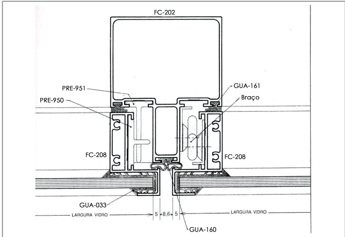
CORTE 04
