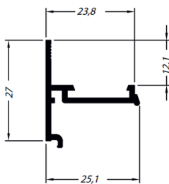
SU292 0,207 Kg/m INVERSOR DE BAGUETE
