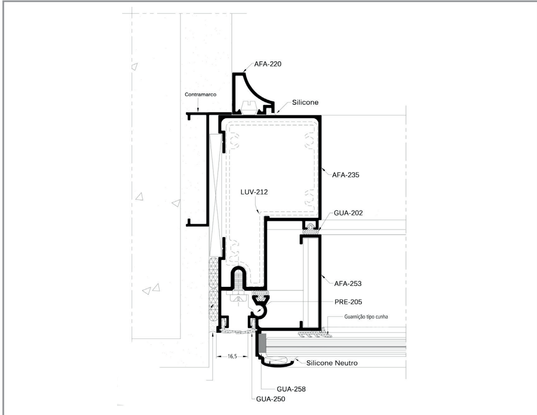
CORTE 04
