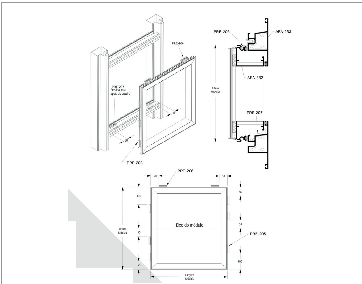
CORTE 06
