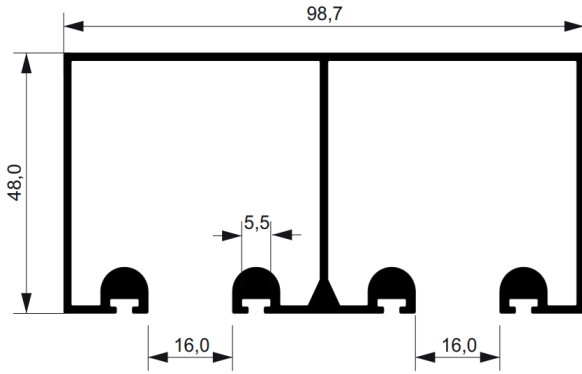
AP38 TRILHO INFERIOR DUPLO 08mm 0,316 Kg/m
