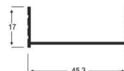
AP - 156 0,184 Kg/m
