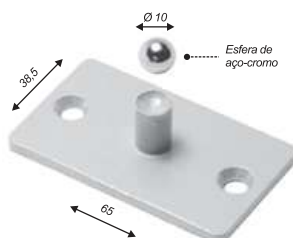
Pivô inferior em inox para 1102
