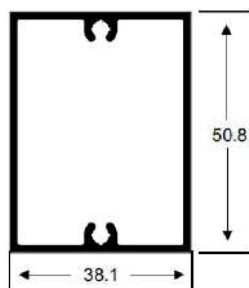
CG - 104 0,802 Kg/m
