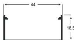
AP - 79 0,316 Kg/m
