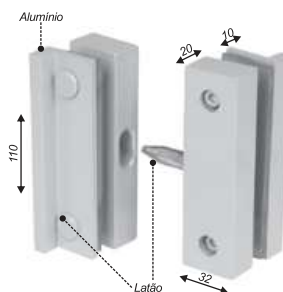
Conjunto mão de amigo para portas de correr com sistema deslizante
