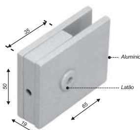
Grapa para sacadas 50x50mm (sem recorte)
