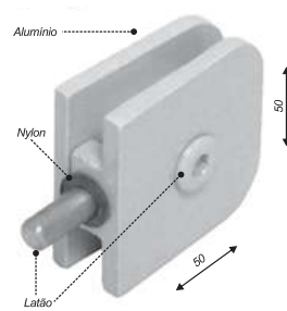
Dobradiça pino para basculante
