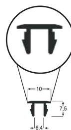
AP - 43 0,079 Kg/m
