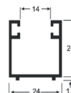
AP - 6 0,345 Kg/m
