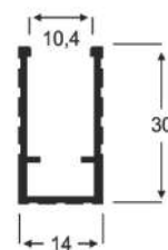
AP - 158 0,192 Kg/m
