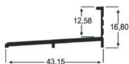
AP - 153 0,173 Kg/m
