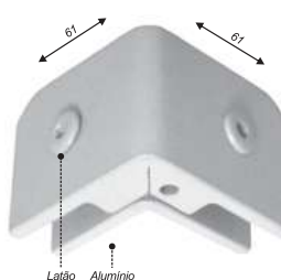
Suporte piso / Teto para união de 2 vidros a 90°
