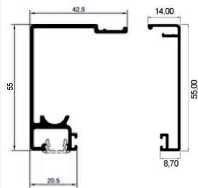
AP - 49A 0,650 Kg/m
