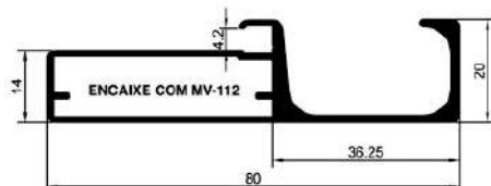
AP-908 0,764 Kg/m
