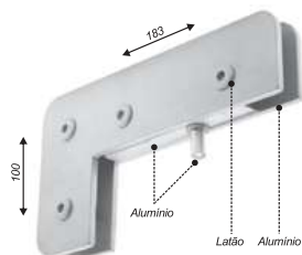
Facão simples para bandeira e fixo
