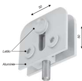
Trinco central para janela e porta de correr
