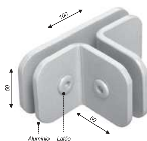
Suporte para união de 3 vidros (sem núcleo)
