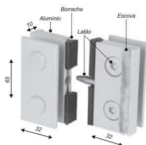
Mini conjunto mão de amigo para sistema 1030
