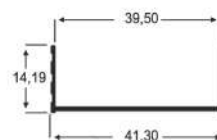
AP - 85 0,164 Kg/m
