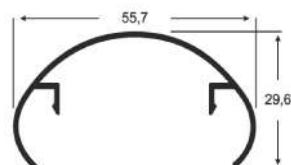
AP - 78 0,417 Kg/m
