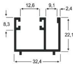
AP - 45 0,357 Kg/m
