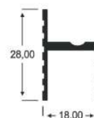
AP - 106 0,228 Kg/m
