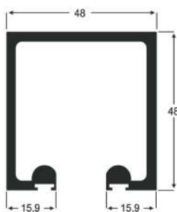
AP - 68 1,209 Kg/m
