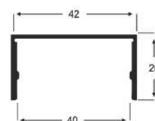
AP - 34 0,241 Kg/m
