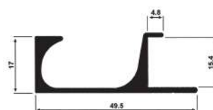
AP-911 0,513 Kg/m
