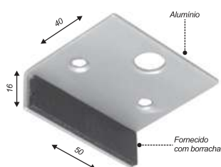
Batedeira para trinco de basculante
