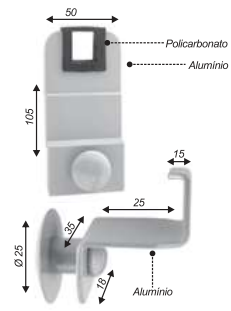
Conjunto acessório V/V para 1587
