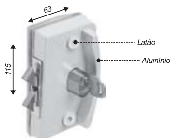
Fechadura direita p/ janela de correr (sem tambor e puxador externo)
