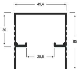
AP - 157 0,580 Kg/m
