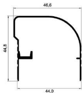
AP - 86 0,447 Kg/m
