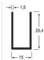
AP - 10 0,210 Kg/m
