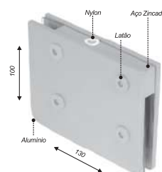
Max dobradiça pivotante superior para portas até 1600mm*
