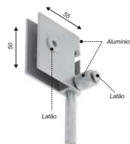
Trinco direito para janela de correr
