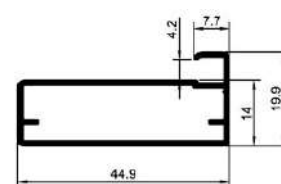
AP-907 0,409 Kg/m
