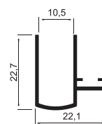
AP - 41 0,000 Kg/m
