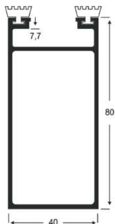
AP - 36 1,207 Kg/m
