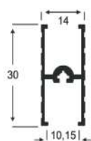
AP - 159 0,214 Kg/m
