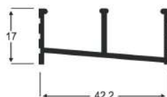
AP - 160 0,226 Kg/m
