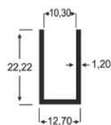
AP - 806 0,181 Kg/m
