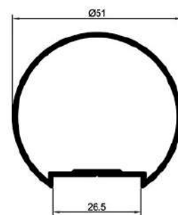
AP - 71 0,675 Kg/m
