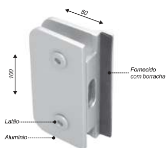
Contra-fechadura V/V com batente para 1520
