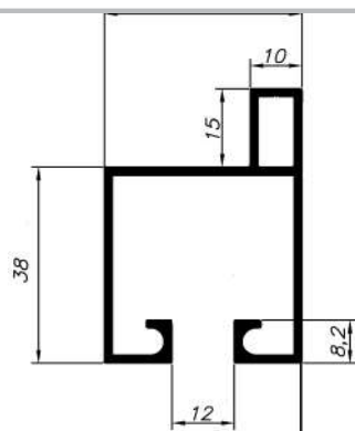
AP - 37A 0,791 Kg/m
