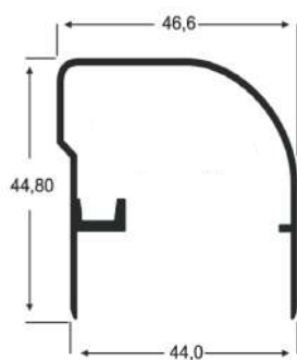
AP - 54 0,450 Kg/m
