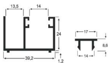
AP - 5 0,411 Kg/m
