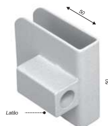
Contratrinco de pressão para 1800C
