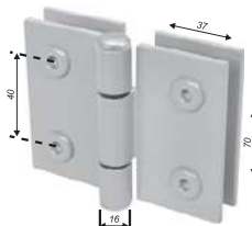
Dobradiça MAXIM-AR V/V (40mm entre furos)
