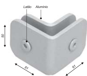
Suporte central para união de 2 vidros a 90°
