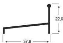
AP - 57 0,184 Kg/m
