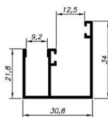
AP - 140 0,365 Kg/m
