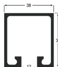
AP - 37 0,728 Kg/m
