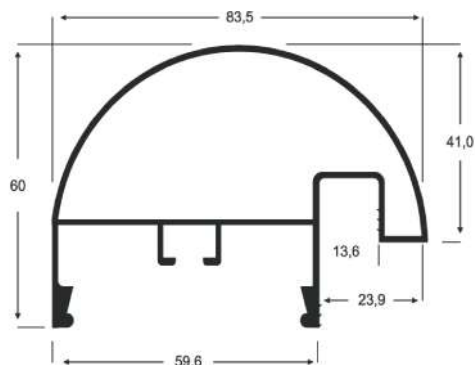
AP - 84 1,098 Kg/m
