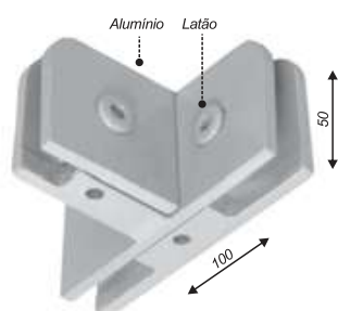
Suporte para união de 3 vidros (com núcleo)
