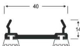
AP - 35 0,376 Kg/m
