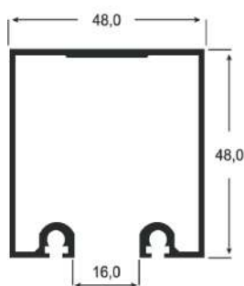
AP - 67 0,881 Kg/m
