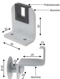
Conjunto acessório V/A para 1587
