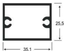
AP - 88 0,622 Kg/m
