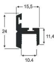
AP - 17 0,260 Kg/m
