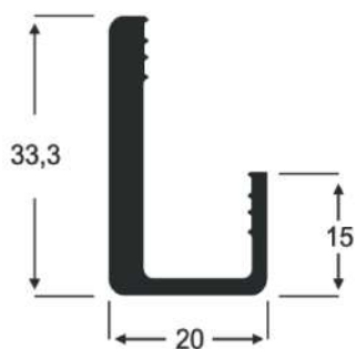
AP - 75 0,558 Kg/m
