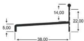
AP - 460 0,189 Kg/m
