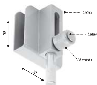
Trinco de pressão sem núcleo
