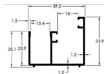
AP - 141 0,458 Kg/m
