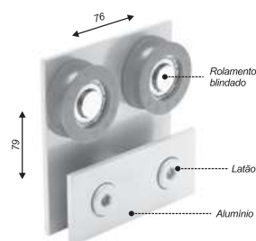
Carrinho duplo 2 furos para AP-68 (portas até 80kg)
