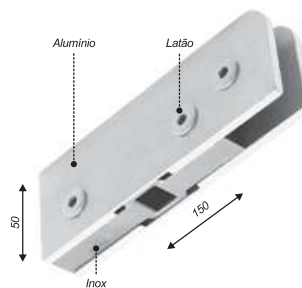
Dobradiça inferior com miolo inox para porta até 1000mm*
