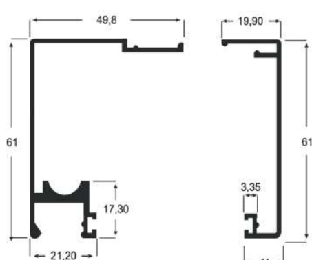
AP - 51A 0,729 Kg/m
