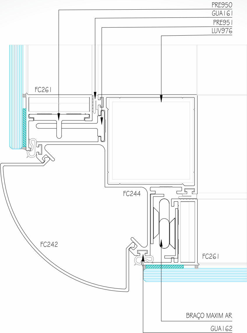
DETALHE CANTO 90°
