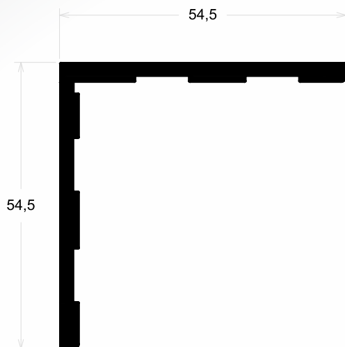
CL007 CANTONEIRA 45° 0,938 Kg/m MEDIDA PADRÃO: 3 METROS
