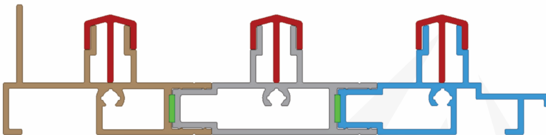
DETALHE APLICAÇÃO VISTA INFERIOR
