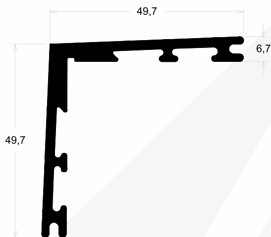
CL006 CANTONEIRA 45° 1,181 Kg/m MEDIDA PADRÃO: 3 METROS
