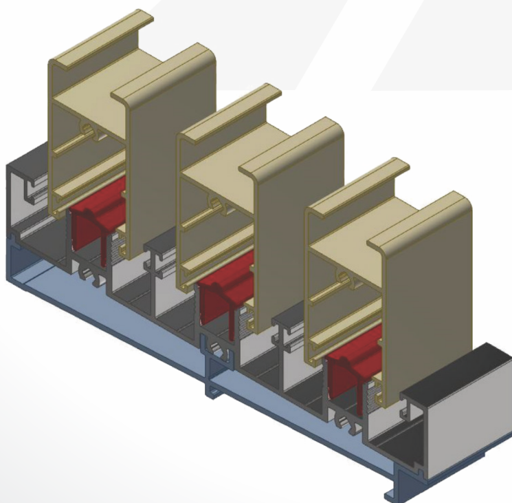
DETALHE APLICAÇÃO VISTA INFERIOR
