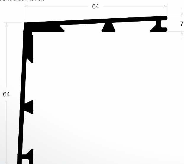
CL044 CANTONEIRA 45° 1,086 Kg/m MEDIDA PADRÃO: 3 METROS
