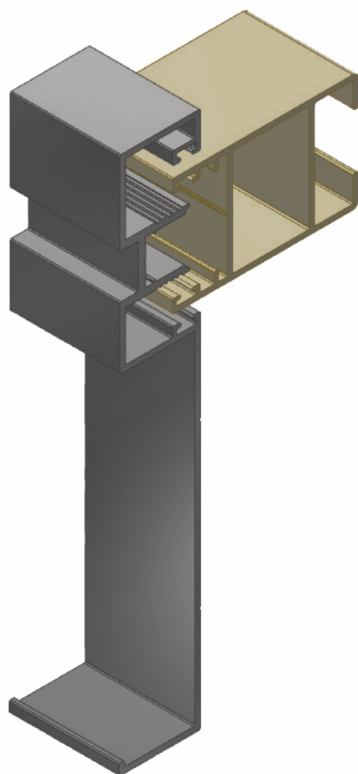
DETALHE APLICAÇÃO VISTA LATERAL
